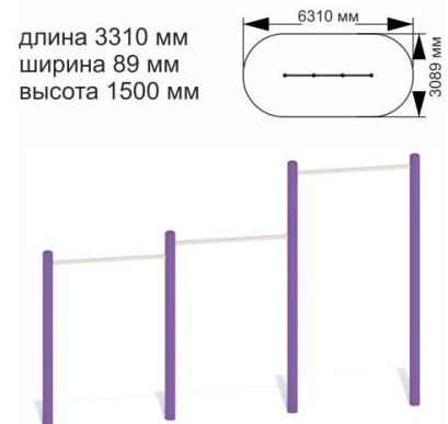
Рис. 6. Турники
