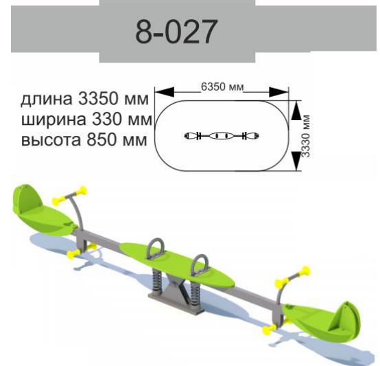
Рис. 4. Качалка-балансир
