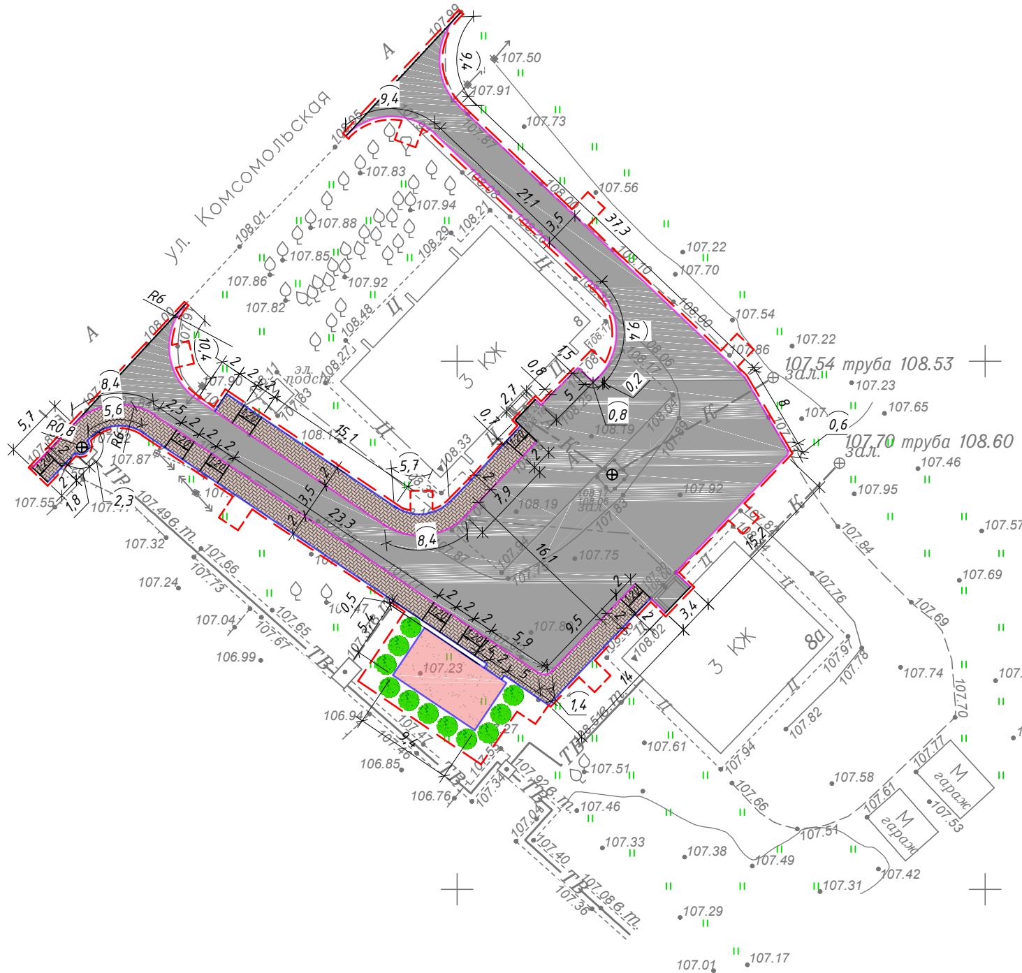
Разбивочный план М1:500
