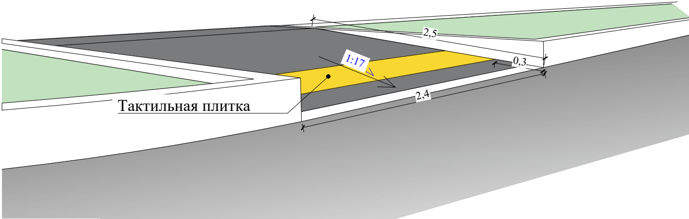
Съезд для МГН тип 1
